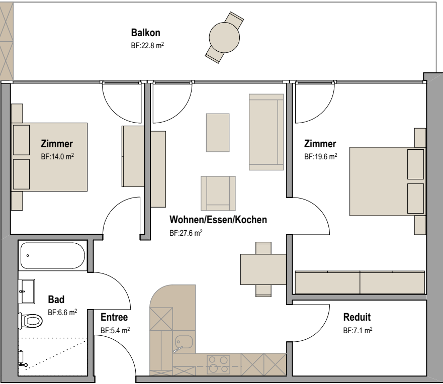
Wohnungsgrundriss Typ 3a
