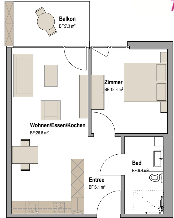
Wohnungsgrundriss Typ 1b
